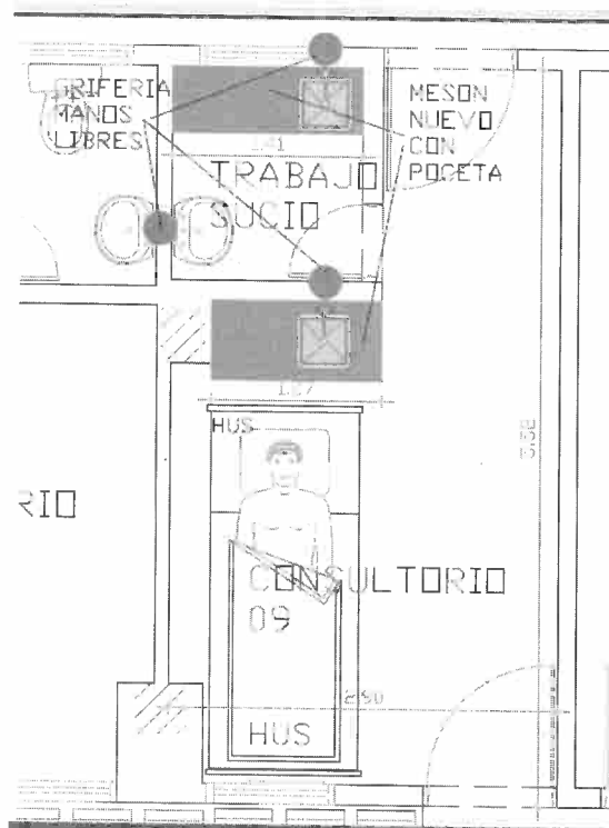
PLANTA CONSULTORIO No 9, PLANTA PROCEDIMIENTOS PARA CONSULTORIOS 16 A, B, C
