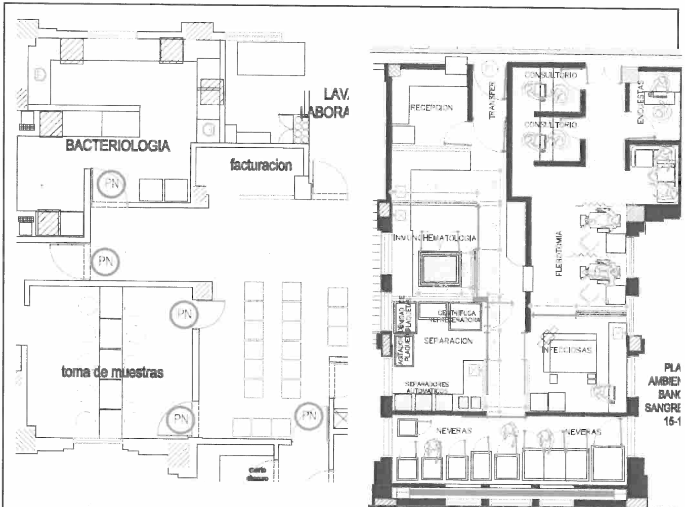
PLANTA HALL LABORATORIOS
