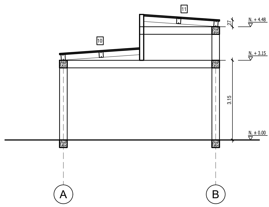
PC ALZADA EJE 4 ESCALA: 1:75
