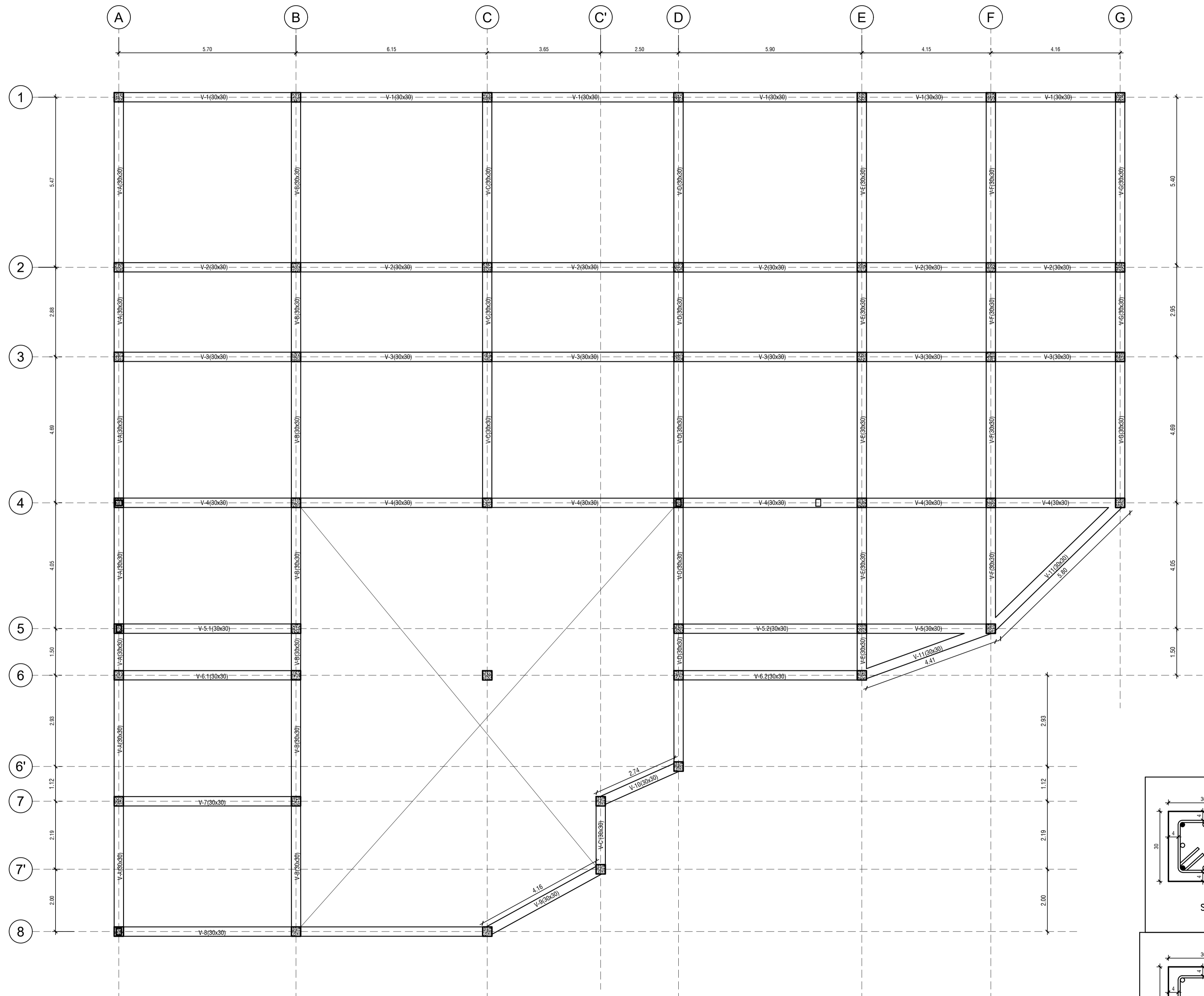
PC1 PLANTA DE VIGAS DE CUBIERTA N+3.15 ESCALA: 1:75
