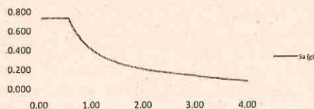
ESPECTRO ELÁSTICO DE DISEÑO Microzonificación Bogotá - NSR-10
